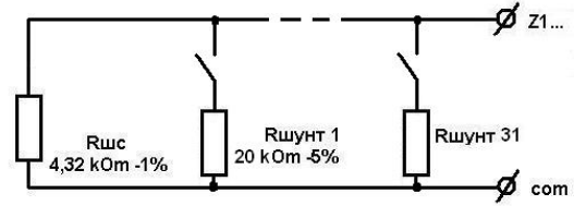
Підключення ШС Z1 ...
