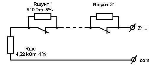
Підключення ШС Z1 ...
