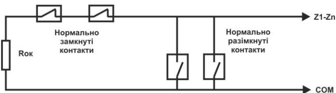
Схема підключення сповіщувачів з нормально замкненими та нормально розімкненими контактами (Мал. 3)
